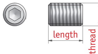
grub screw (DSG)
